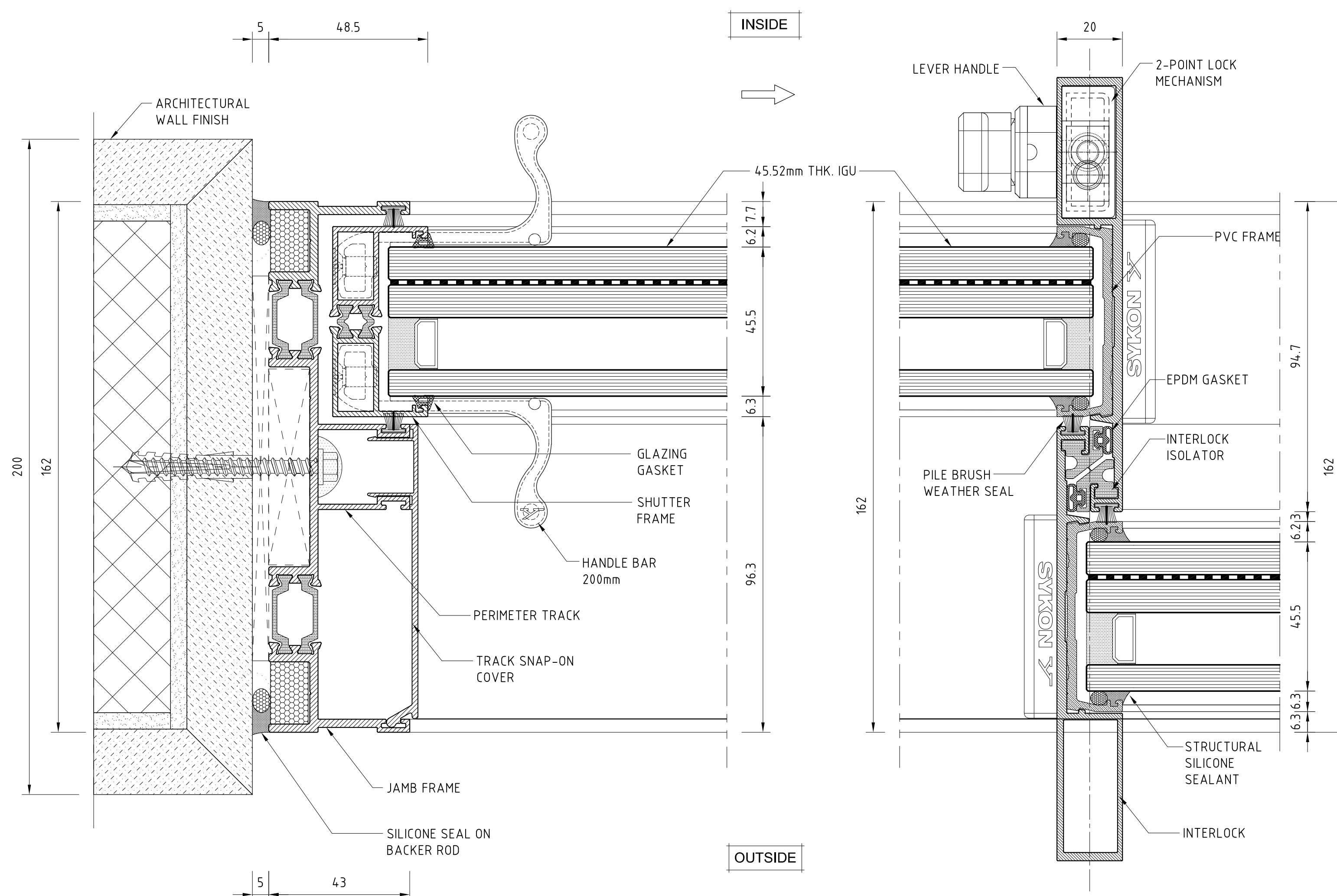
JAMB DETAIL
